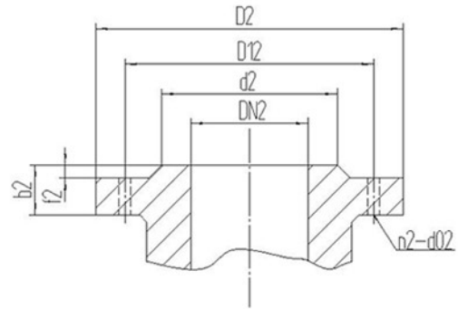
Outlet Flange Data
